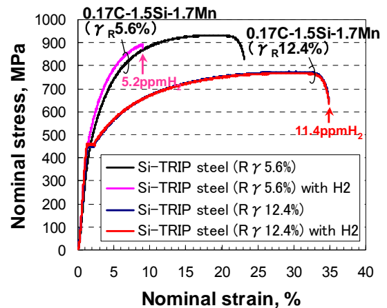
図3 Si系TRIP鋼( \gamma_R=5.6\% 、 12.4\% )の引張変形挙動に及ぼす水素の影響
