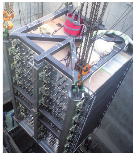
⑤ ビームダンプ ビームライン下流にはグラファイトブロックを用いたビームダンプが設置されています。ニュートリノ以外の粒子はこのビームダンプに吸収されます。
