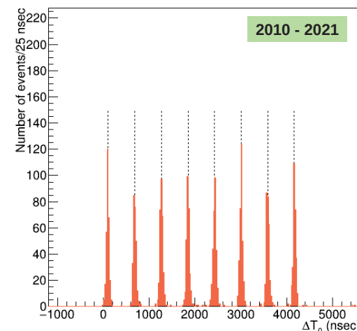
ニュートリノ事象の時間分布。 ニュートリノビームの 8 パンチ構造が 確認できる。
