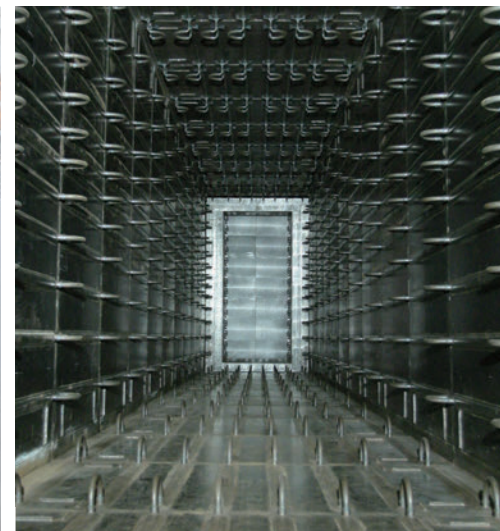
④ ディケイボリューム パイ中間子は約 100m のディケイボリュームで崩壊し、ニュートリノが生成されます。
