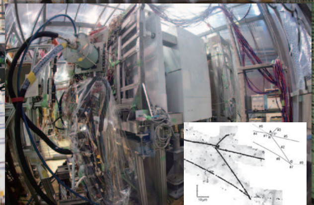
KURAMA スペクトロメータと発見された「美濃イベント」
